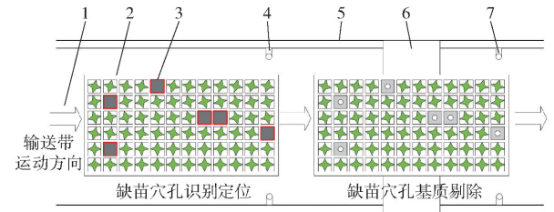
图 2 气吸式基质剔除装置作业原理图
