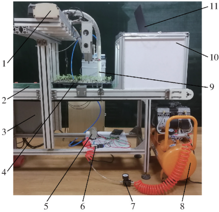
图 13 气吸式基质剔除试验平台
