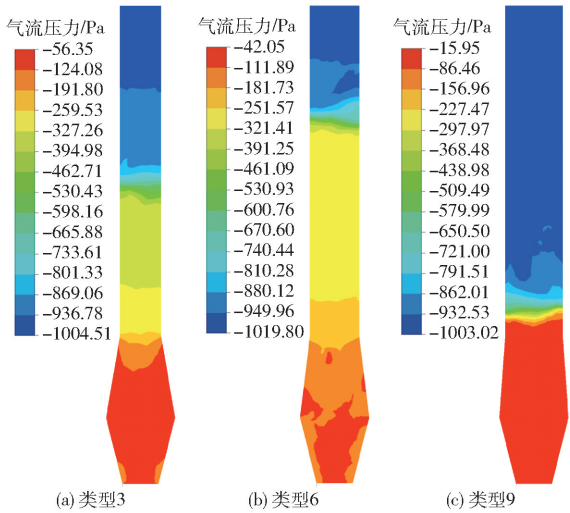
图 8 气流压力分布云图
