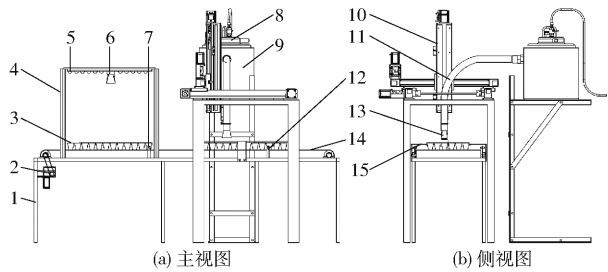
图 1 气吸式基质剔除装置结构简图
