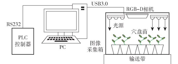
图 10 穴盘缺苗识别系统
