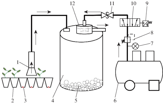
图3 气流输送系统示意图
