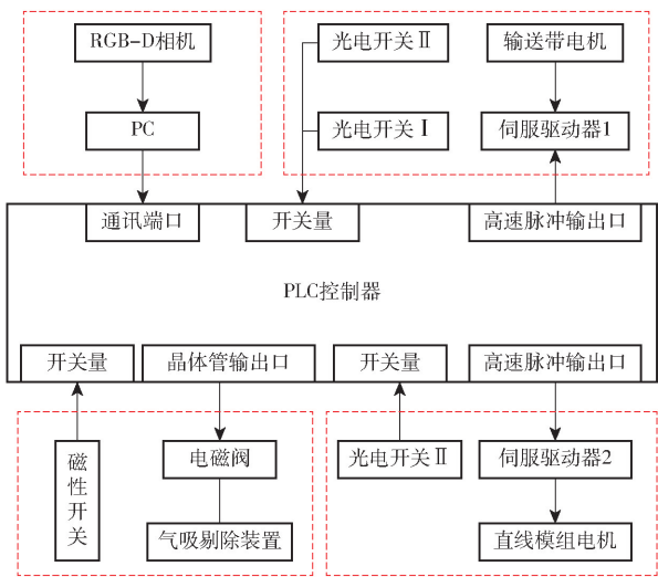
图 12 控制系统原理图
