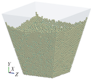
图 6 基质仿真模型 Fig. 6 Simulation model of substrate
