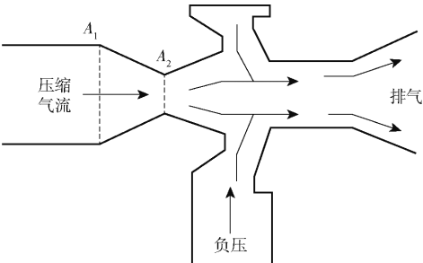
图4 负压产生原理图
