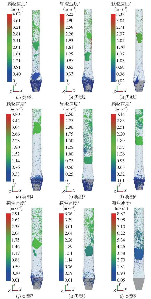
图 7 基质剔除过程
