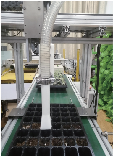
图 14 气吸式基质剔除测试
