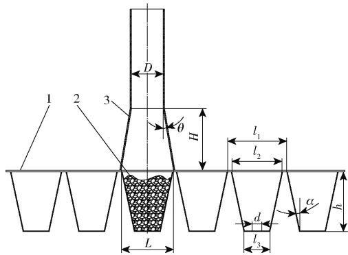
图 5 气吸端口结构示意图
