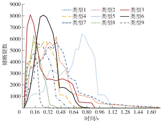
图 9 基质键断裂数变化曲线
