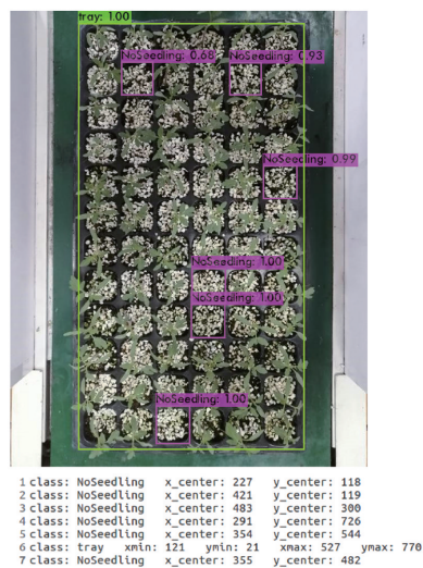
图 11 缺苗穴孔识别与定位结果
