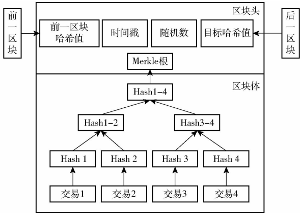
图 2 区块结构图 Fig. 2 Structure diagram of block
