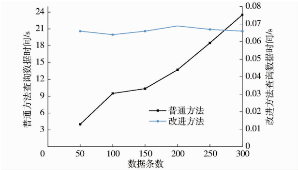
图5 普通方法和改进方法在不同数据条数下查询数据时间对比
