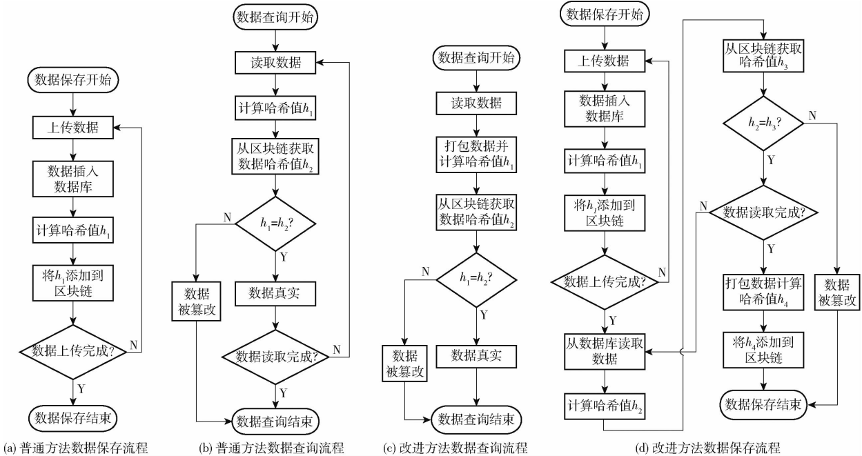
图 3 普通方法和改进方法试验流程图 Fig. 3 Test flow charts of common method and improved method
