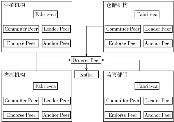
图6 Fabric 系统结构图
