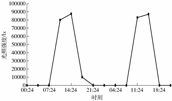
图 8 物联网平台数据检测曲线
