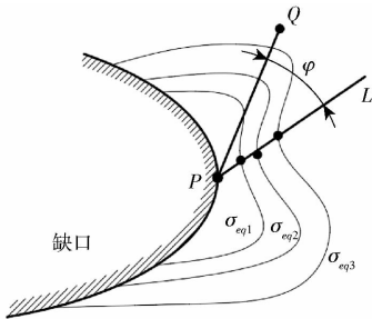
图 1 应力梯度方向角确定方法
