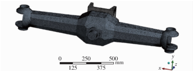
图 3 转向驱动桥壳有限元模型
