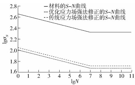
图 14 转向驱动桥壳结构 S-N 曲线修正
