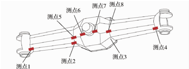
图 5 转向驱动桥壳测点示意图
