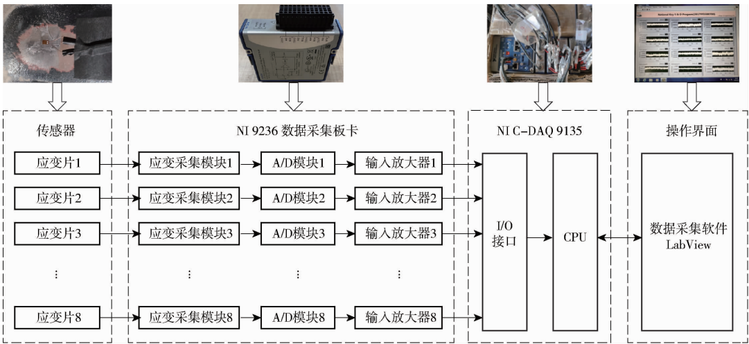
图 6 动态载荷测试采集系统示意图
