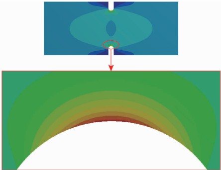
图 12 U 形缺口试件应力分布云图
