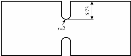
图 11 U 形标准缺口试件示意图
