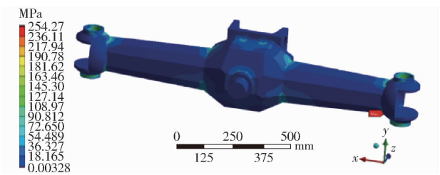
图 4 转向驱动桥壳应力云图
