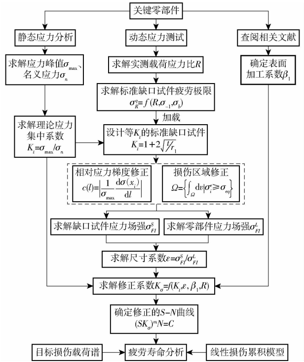
图 2 基于田间实测载荷的疲劳寿命分析技术路线图
