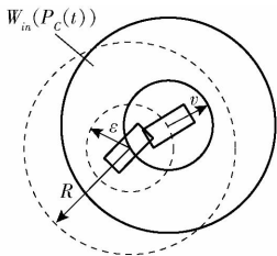
图 2 滚动窗口算法原理图
