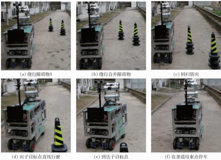
图 16 AGV 连续绕行 2 个小间距静态障碍物的避障试验过程
