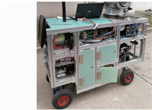
图 14 AGV 试验系统
