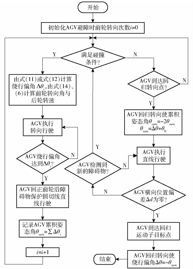
图 11 调节 \Delta\theta 的避障算法流程图
