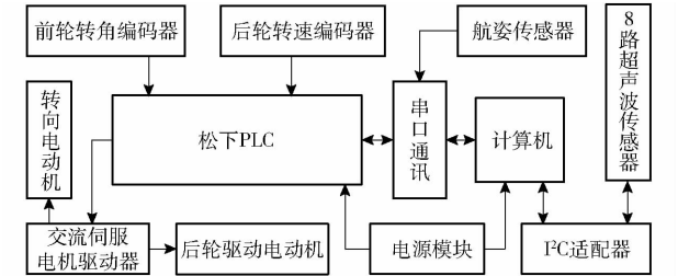
图 12 AGV 控制系统硬件组成
