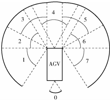
图 3 8 路超声波传感器配置方案
