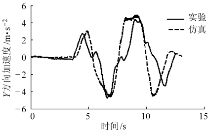
图 4 实验加速度与仿真加速度对比
