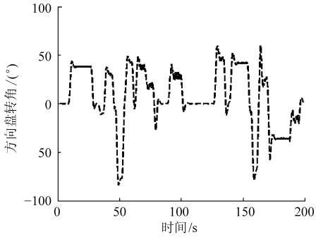
图 8 复杂路况转向盘转角 (40 km/h)
