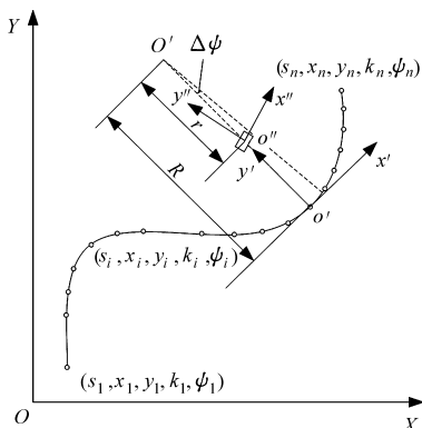
图 1 道路信息描述
