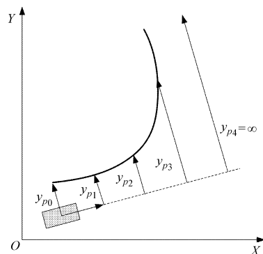
图 2 依据车辆坐标方向预瞄
