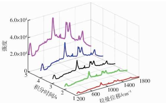
图 4 不同积分时间对猪肉中莱克多巴胺 SERS 光谱的影响
