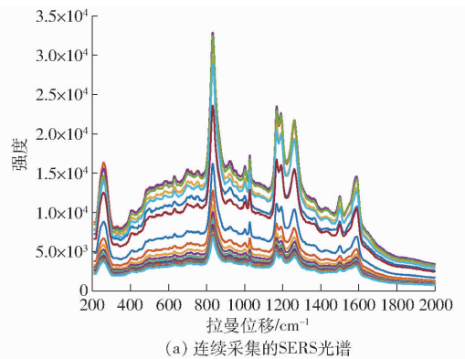
(a) 连续采集的 SERS 光谱
