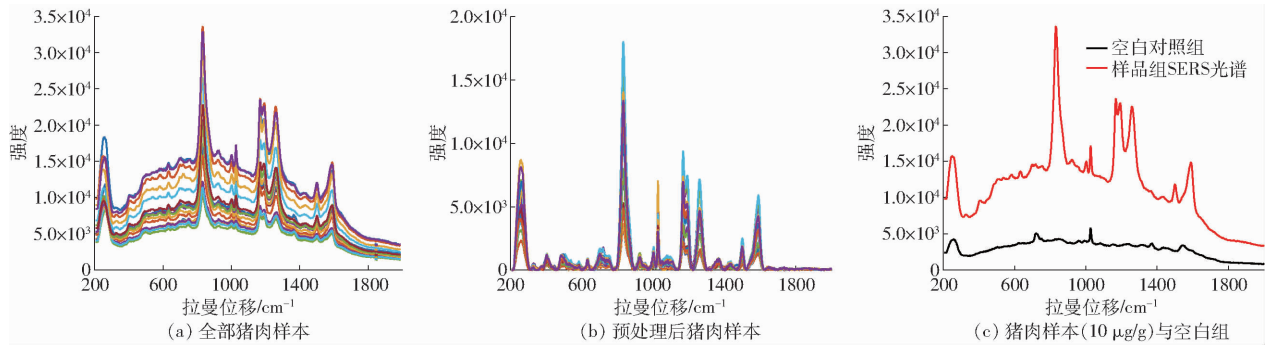
图 3 猪肉样本的 SERS 光谱
