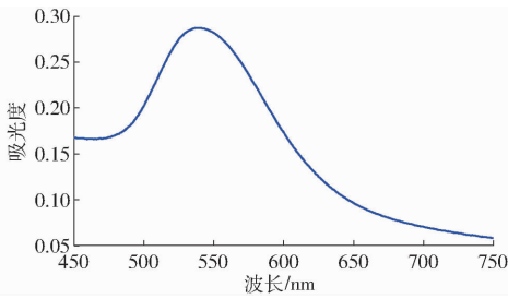
图 2 金溶胶的紫外可见吸收光谱
