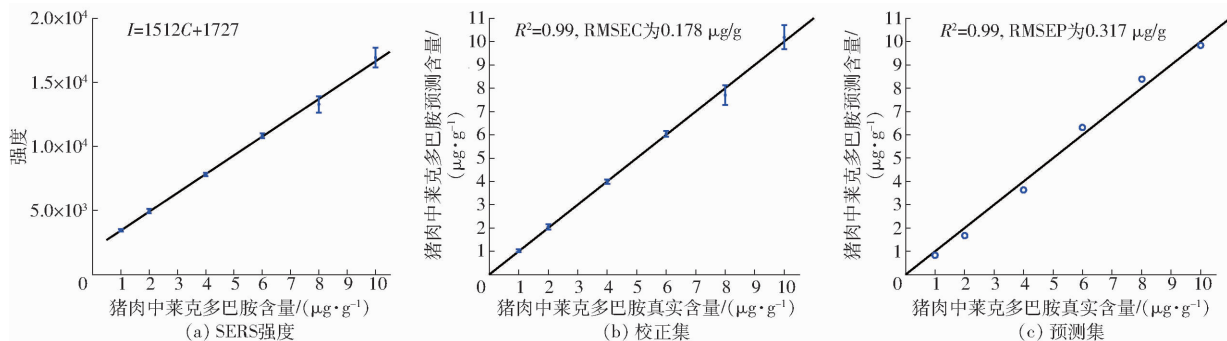
图9 猪肉中莱克多巴胺在 831 cm -1 处 SERS 强度以及预测浓度与真实浓度的关系
