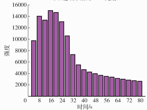
(b) 831 cm -1 处强度随时间变化
