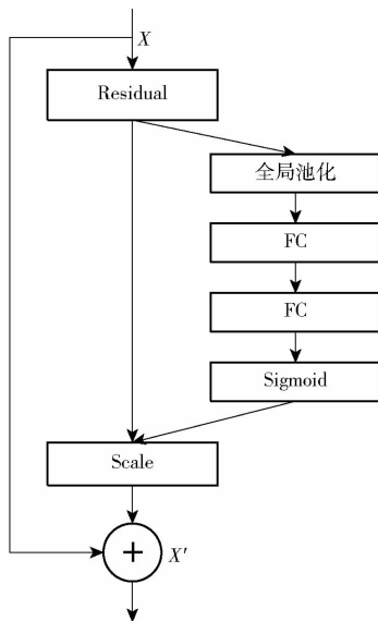
图4 SE-ResNet 模块
